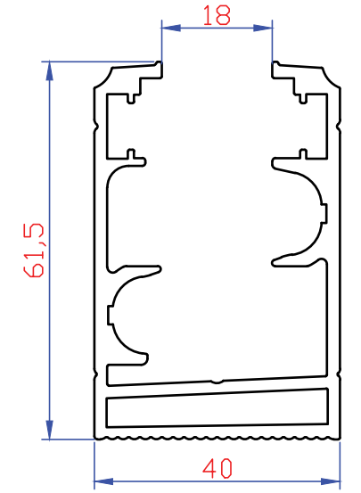
2413 1528 gr/mt Pelit Üst Kasa
