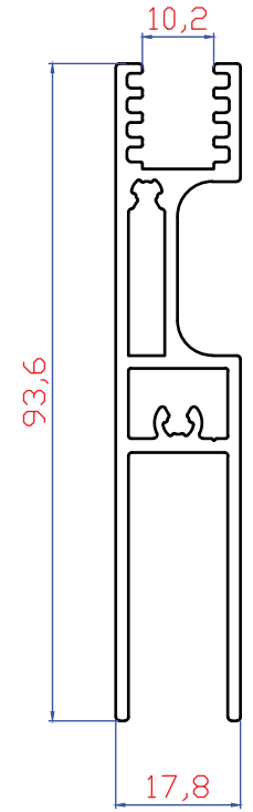
2320 1279 gr/m Alt Baza 10 mm
