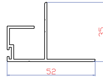
8503 473 gr/mt Fotosel Çıtası
