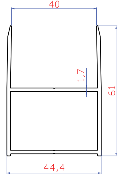
2048 924 gr/mt Üst Ayar Profili
