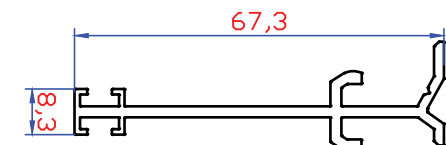
2575 588 gr/mt Yan Dikme Ara Kılavuz
