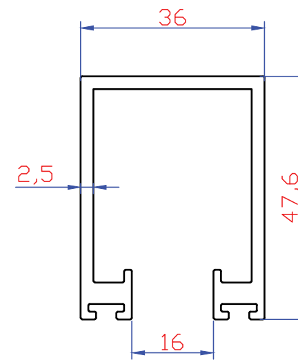
2585 1078 gr/mt Kapi Kanat B
