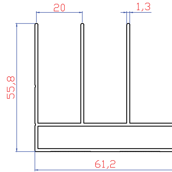
2414 1102 gr/m 3'lü Sürme Üst Kasa
