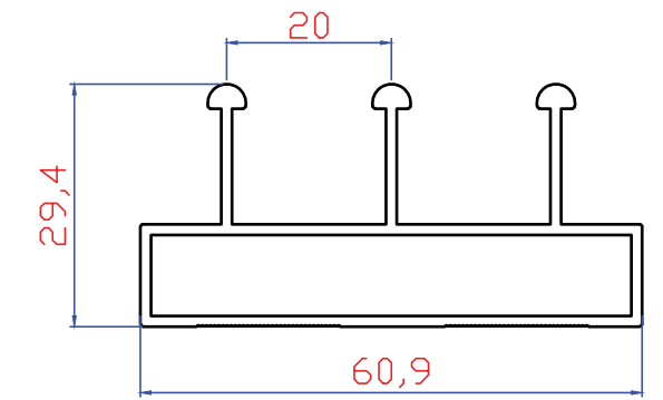
2416 735 gr/m 3'lü Sürme Eşikli Alt Ray
