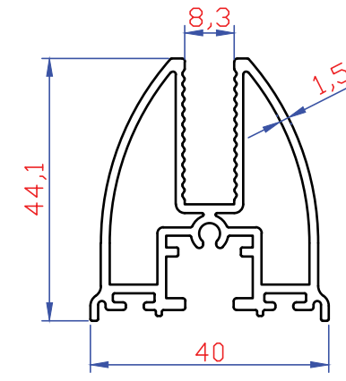
2258 959 gr/mt Firtina Baza 8 mm
