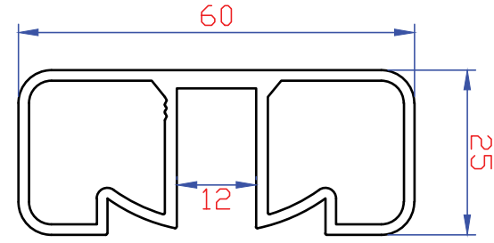
2777 933 gr/m 60x25 Ortadan Camlı Profil
