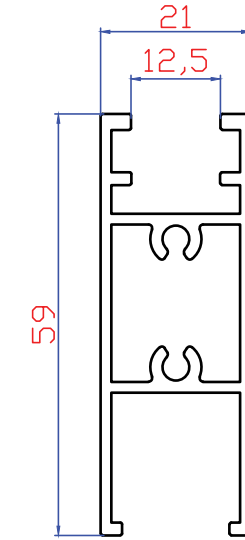
8502 799 gr/mt Üst Etek
