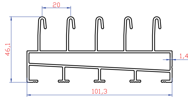
8478 1.813 gr/m Eşikli Alt Ray
