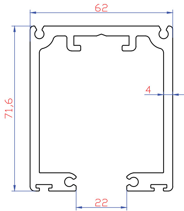
2933 2872 gr/m Kasa Profili
