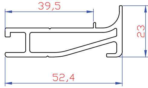
2156 770 gr/mt Alt Su Tahliye Profili
