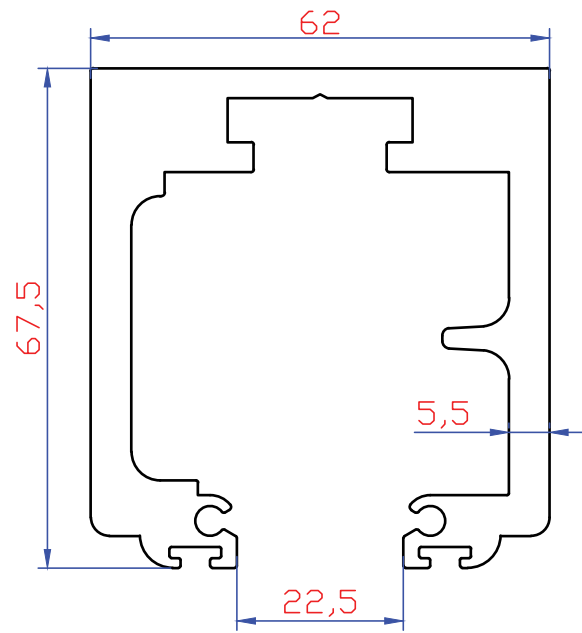
2704 3916 gr/m Kasa Profili
