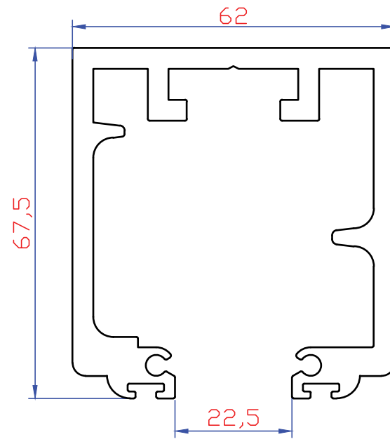
2587 2988 gr/mt Kasa Profili
