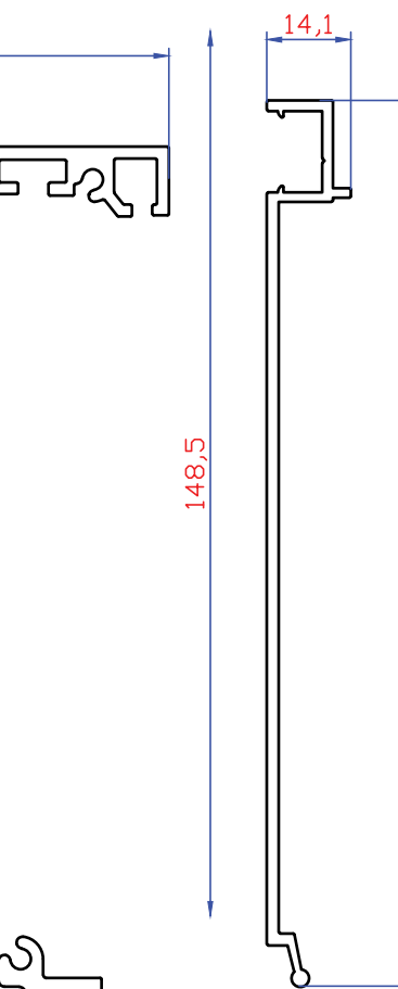
8578 911gr/m Şase Kapak
