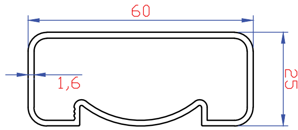
2778 713 gr/m 60x25 Camsız Profil
