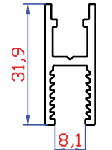
2695 394 gr/mt Dikey Baza 8 mm
