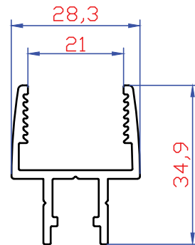
2752 511 gr/mt Dikey Baza 21 mm
