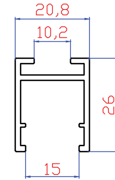
8504 335 gr/mt U Çıta
