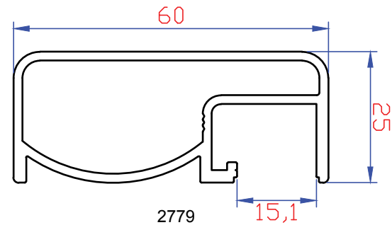
2779 888 gr/m 60x25 Önden Camlı Profil
