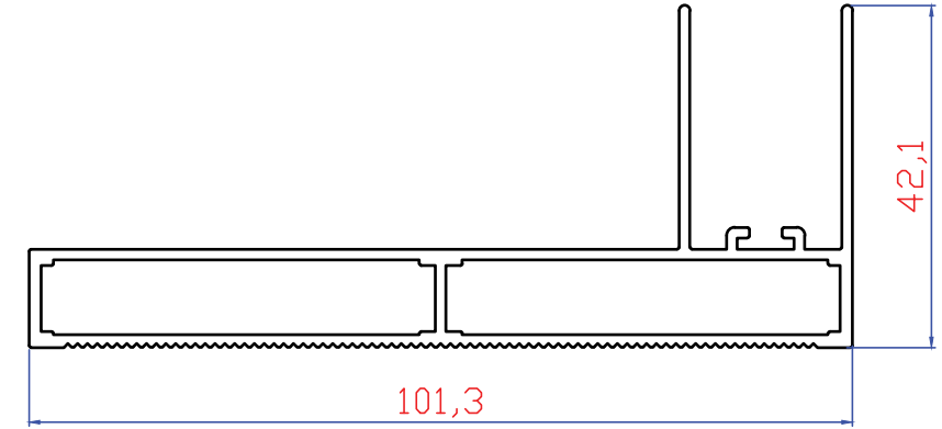
2322 1110 gr/m Yan Kasa
