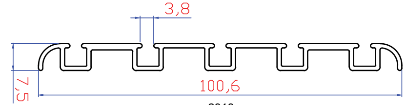
2318 634 gr/m Eşiksiz Alt Ray
