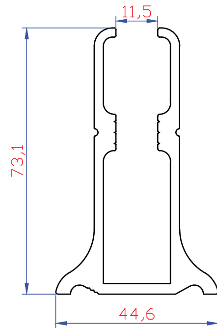
2781 1725 gr/m A/F Baza Profili
