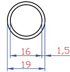
1512 223 gr/m 19'luk Boru
