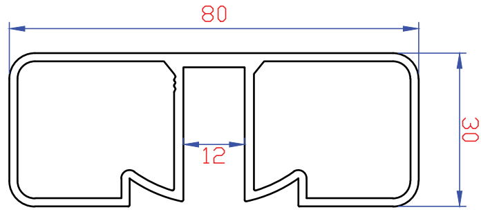
2776 1199 gr/m 80x30 Ortadan Camlı Profil
