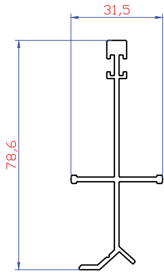
2747 643 gr/mt Yan Dikme Ara Kılavuz
