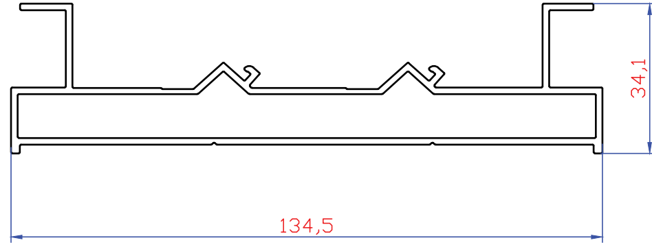
2746 1487 gr/mt Yan Dikme
