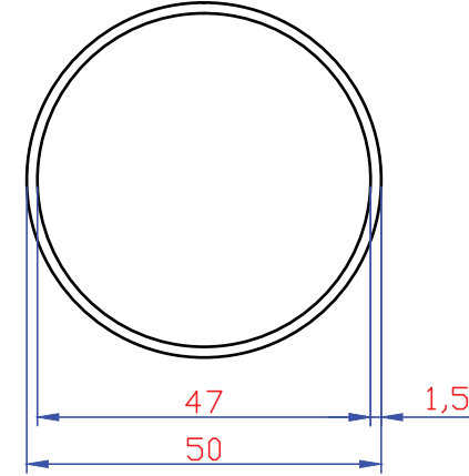
1527 619 gr/m 50'lik Boru
