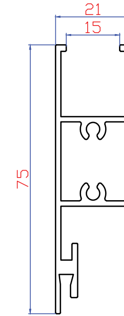
8501 966 gr/mt Alt Etek
