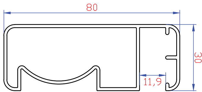
8477 967 gr/m 80x30 Önden Camlı Profil EKO
