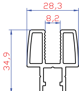
2751 666 gr/mt Dikey Baza 8 mm
