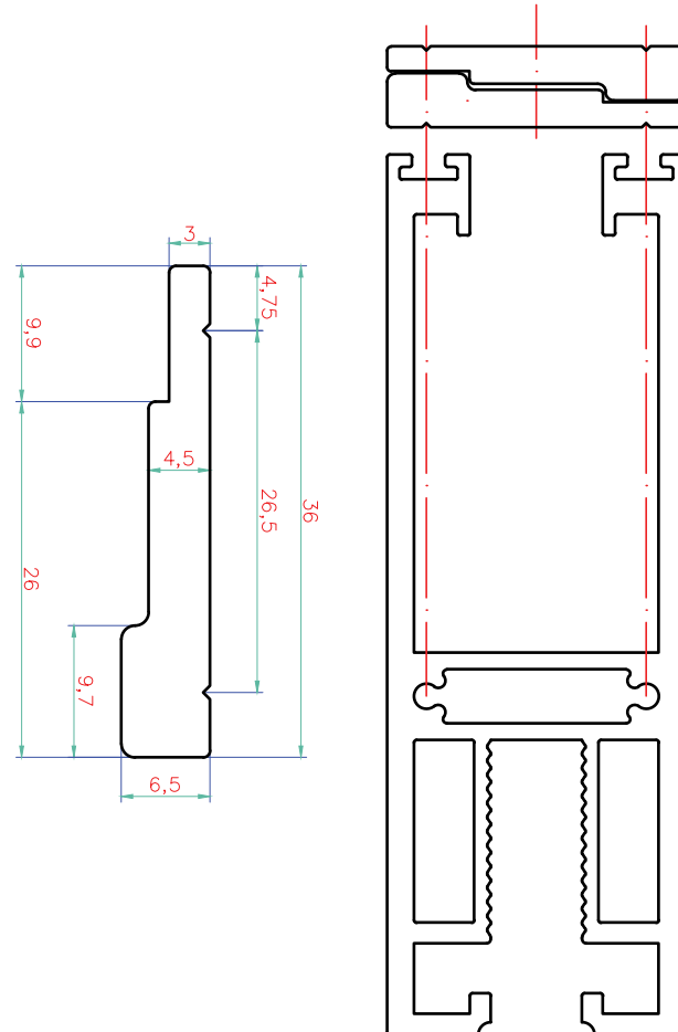
2587 2988 gr/mt Kasa Profili
