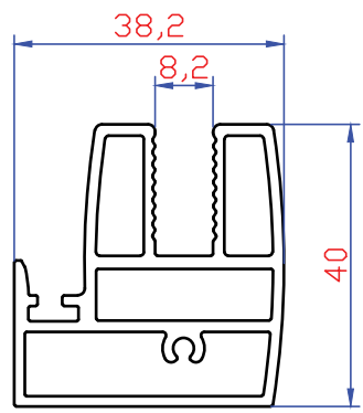
2750 1054 gr/mt Yatay Baza 8 mm
