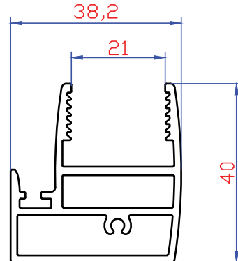
2749 911 gr/mt Yatay Baza 21 mm
