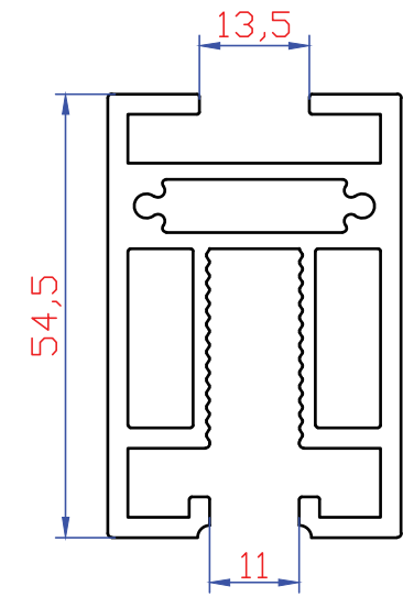
2586 1805 gr/mt Kapi Kanat A
