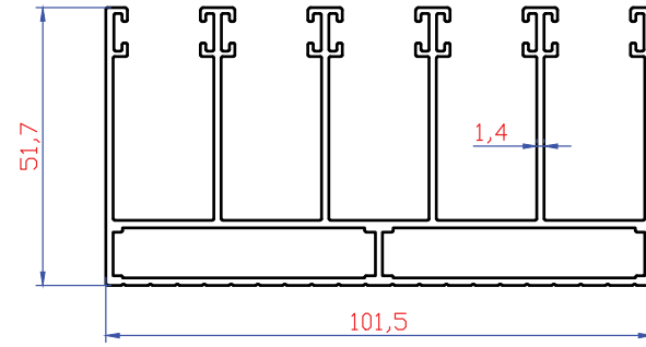
8479 1.994 gr/m 5'li Sürme Üst Kasa
