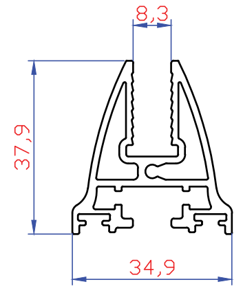
2394 R1 851 gr/mt Pelit Baza
