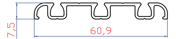
2415 398 gr/m 3'lü Sürme Eşiksiz Alt Ray
