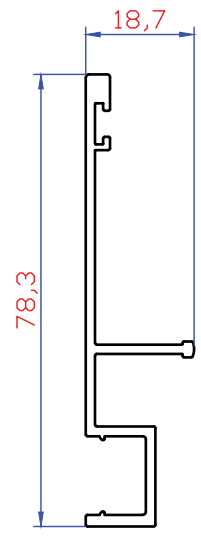
2748 579 gr/mt Yan Dikme Kapak
