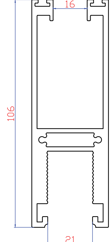
2729 2830 gr/mt Kanat 21 mm
